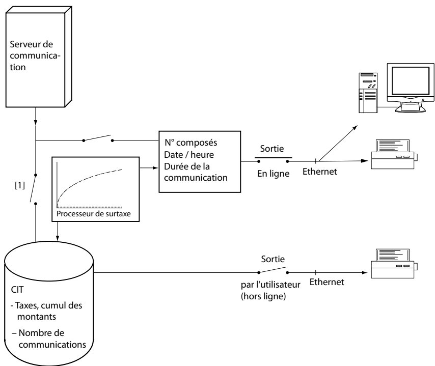
Fig. 133 Observation du trafic et enregistrement des données de taxe du trafic sortant
