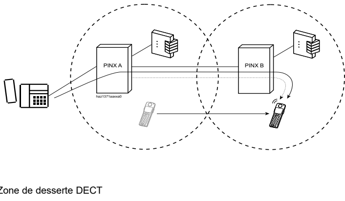
Fig. 196 Activation automatique de DECT Follow me
