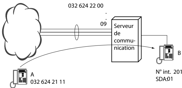
Fig. 161 Appel à un utilisateur libre suivi d'une conversation
