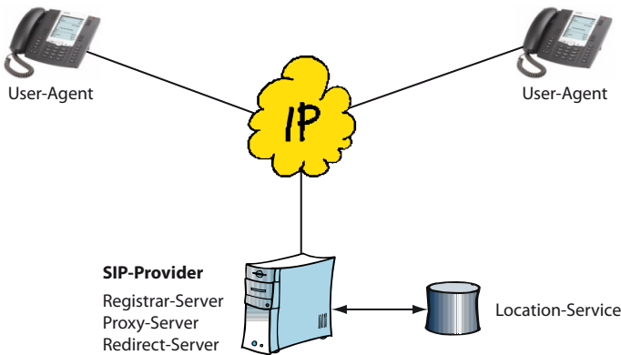
Fig. 11 Composants SIP
