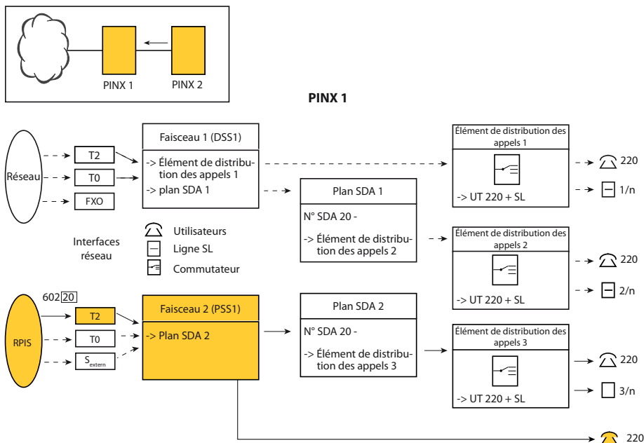
Fig. 87 Acheminement d'un appel depuis le réseau privé fixe sans sélection directe à l'arrivée
