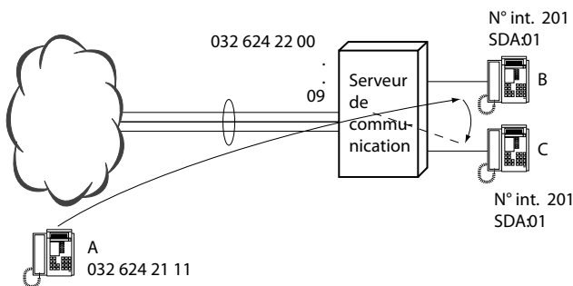
Fig. 166 Communication commutée
