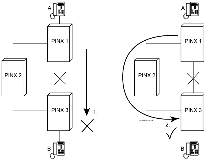
Fig. 122 Routage de débordement dans le réseau privé fixe via des lignes permanentes
