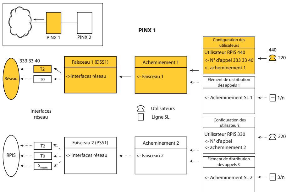
Fig. 96 Acheminement d'un appel à un utilisateur RPIS en réseau virtuel via le réseau public
