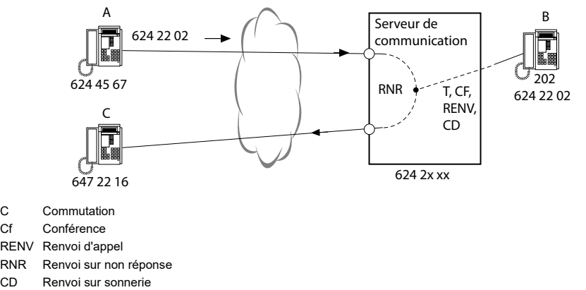
Fig. 109 Connexion réseau-réseau
