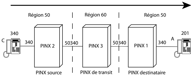
Fig. 42 Exemple 2 : L'utilisateur C appelle l'utilisateur A, acheminement de débordement (détail de la Fig. 40)
