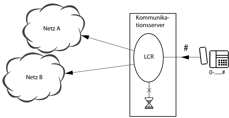
Fig. 212 Numérotation avec caractère de fin de numérotation et fonction LCR active
