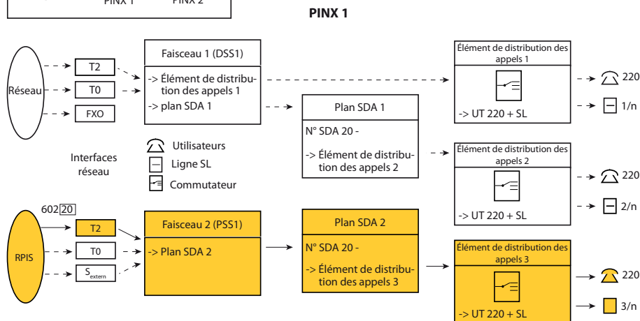
Fig. 86 Acheminement d'un appel depuis le réseau privé fixe avec sélection directe à l'arrivée
