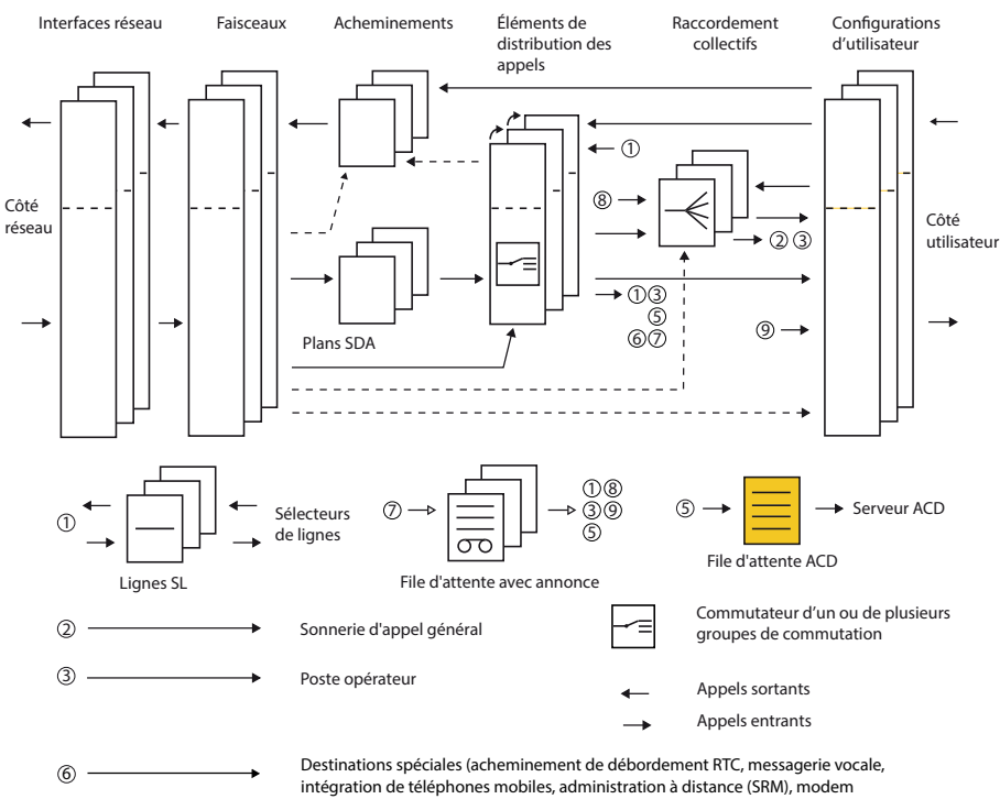
Fig. 78 Le serveur ACD par rapport aux autres éléments de routage
