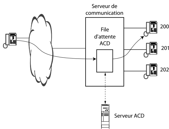
Fig. 79 Routage des appels du serveur de communication piloté par le serveur ACD
