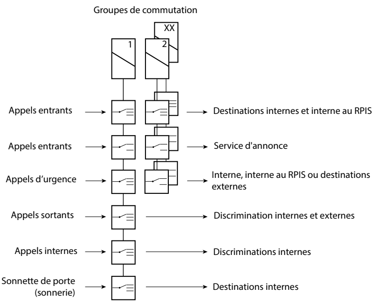
Fig. 62 Les groupes de commutation et la mise en œuvre de leurs commutateurs
