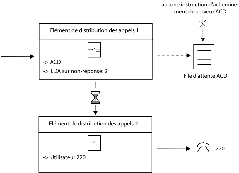
Fig. 80 Acheminement de secours en cas de panne du serveur ACD
