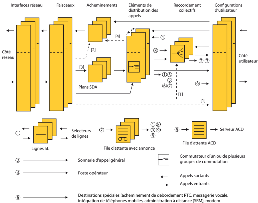
Fig. 49 Le routage des appels dans le système
