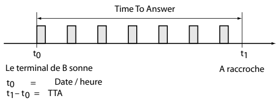
Fig. 164 Durée de la phase d'appel TTA
