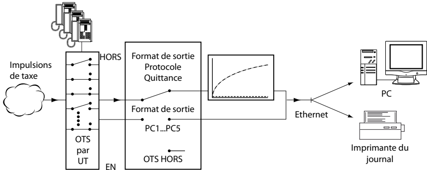
Fig. 147 Déroulement schématique
