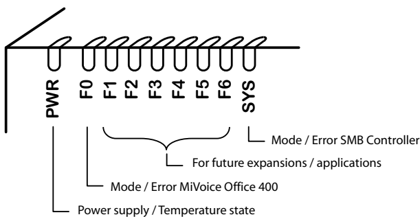
Fig. 74 LED-display
