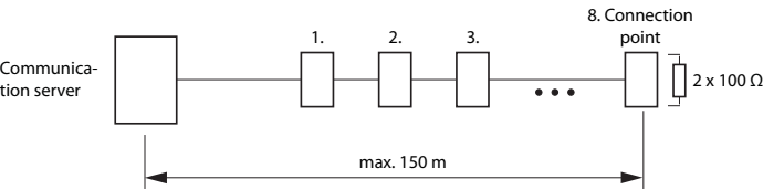
Fig. 45 S-bus, kort
