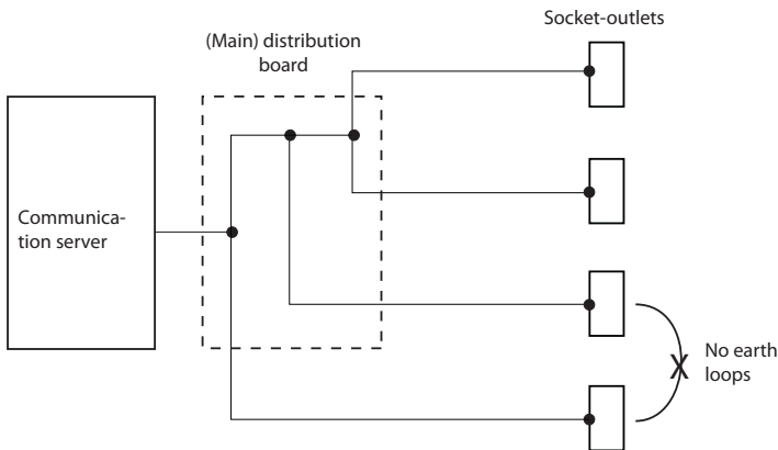
Fig. 20 Boomstructuurprincipe
