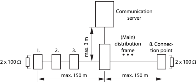
Fig. 46 S-bus, kort, V-vormig
