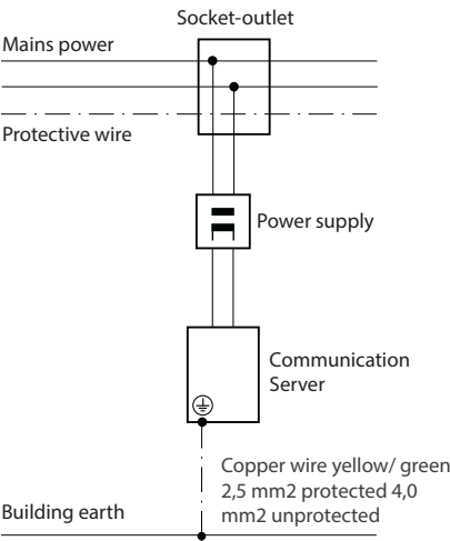
Fig. 19 Aarding van de communicatieserver in het geval van een indirecte bekabeling en een directe bekabeling
