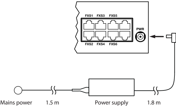
Fig. 21 De communicatieserver voeden vanuit het stroomnet
