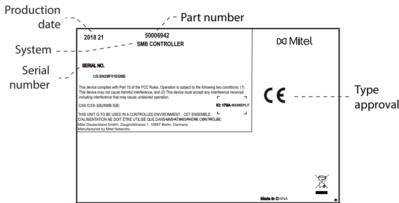
Fig. 78 Typeplaatje Mitel SMB communicatieserver
