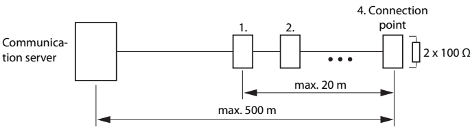
Fig. 47 S-bus, lang
