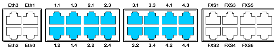
Fig. 39 Aansluitmogelijkheden voor DSI eindstationinterfaces op afzonderlijk toegewezen RJ45 aansluitpunten
