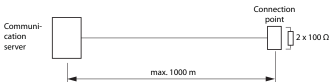
Fig. 48 S-bus, punt-naar-punt
