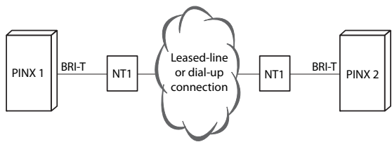
Fig. 32 Basissnelheid-interface BRI-T, in een netwerk met gehuurde lijnen of kiesverbinding
