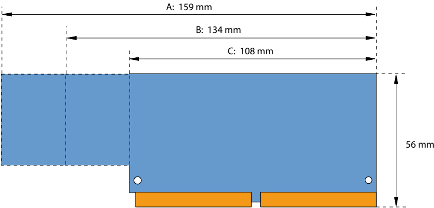
Fig. 80 Afmetingen van interfacekaarten (ontwerp A, B, C)
