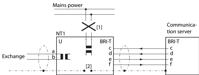
Fig. 30 Basale toegang op NT1
