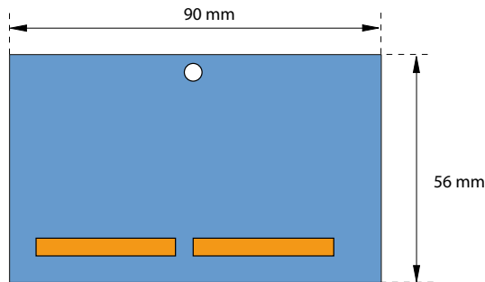
Fig. 81 Afmetingen van systeemmodule (ontwerp D)
