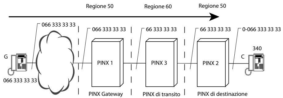
Fig. 47 Esempio 7: L'utente G chiama l'utente C attraverso il PINX 3 (dettaglio della Fig. 40)
