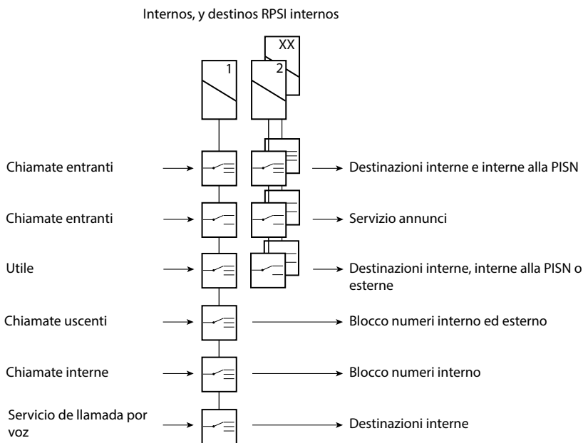
Fig. 62 I gruppi servizi e le funzioni dei commutatori di posizione
