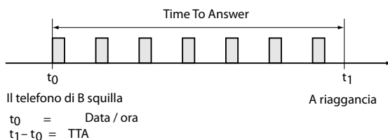
Fig. 164 Durata TTA della fase di segnalazione della chiamata
