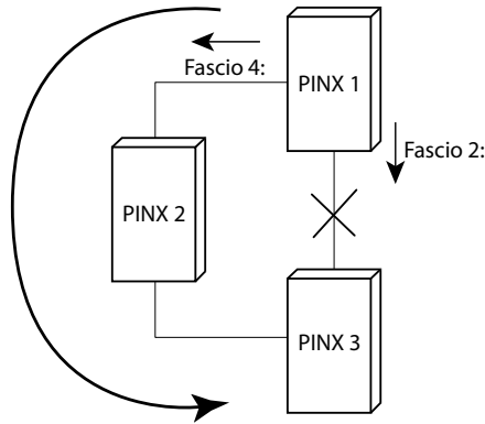
Fig. 123 Instradamento di traffico nella rete privata fissa mediante l'attribuzione di fasci validi nella configurazione dell'instradamento
