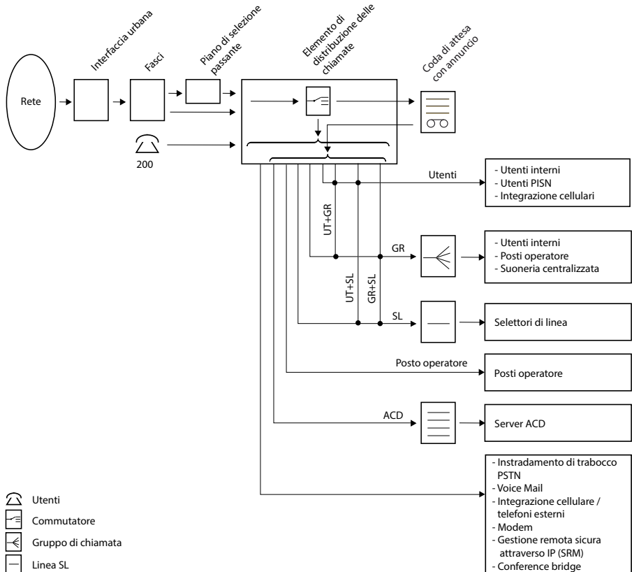
Fig. 58 Destinazioni dell'Elemento di distribuzione delle chiamate
