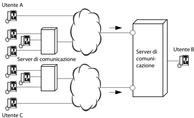
Fig. 112 Collegamento di due chiamate entranti
