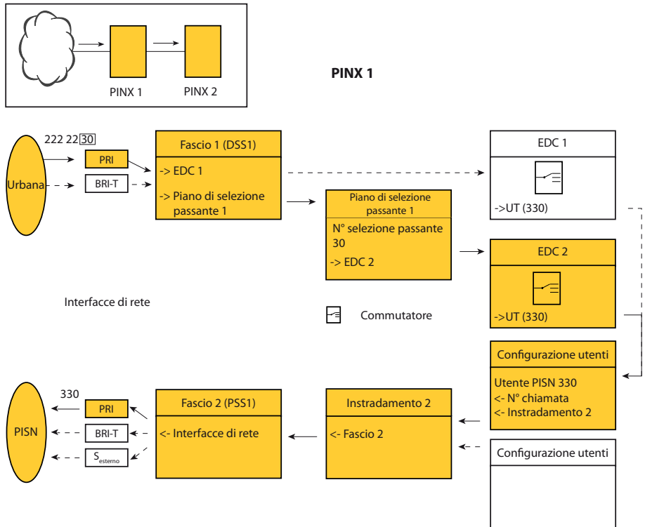
Fig. 117 Instradamento di transito dalla rete pubblica alla rete privata fissa con selezione passante
